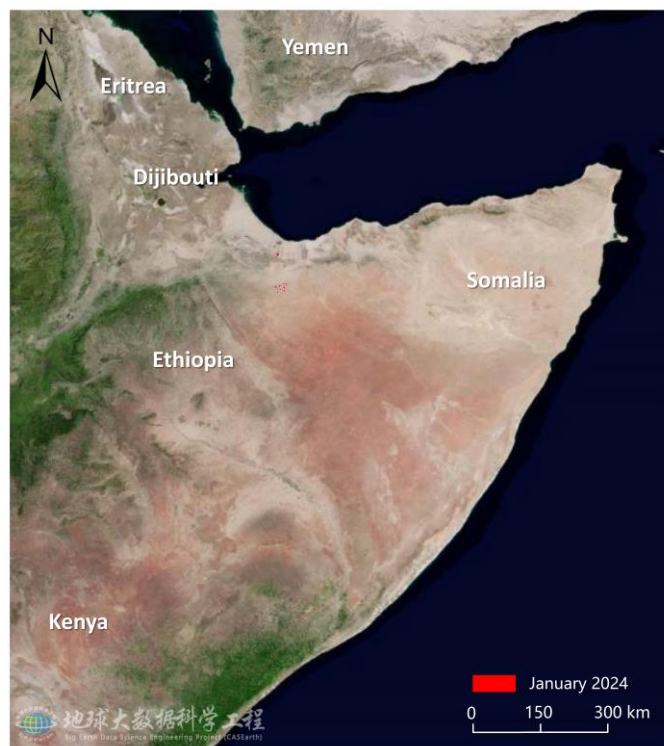
图 3. 索马里沙漠蝗危害区域遥感监测图（2024 年 1 月）
