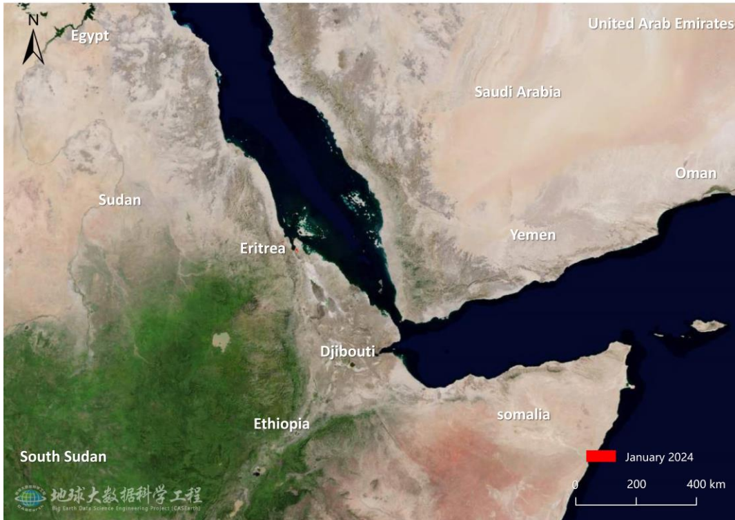
图 2. 厄立特里亚沙漠蝗危害区域遥感监测图 (2024 年 1 月)
