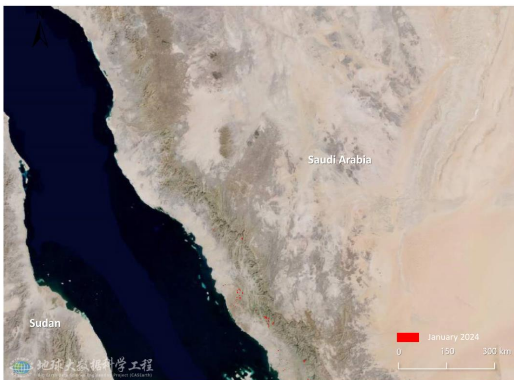
图 1. 沙特阿拉伯沙漠蝗危害区域遥感监测图（2024年1月）
