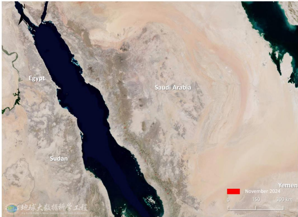
图 3. 沙特阿拉伯沙漠蝗危害区域遥感监测图（2024 年 11 月）
