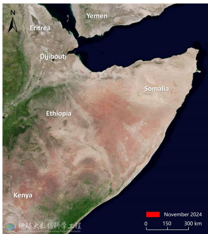
图 2. 索马里沙漠蝗危害区域遥感监测图（2024 年 11 月）
