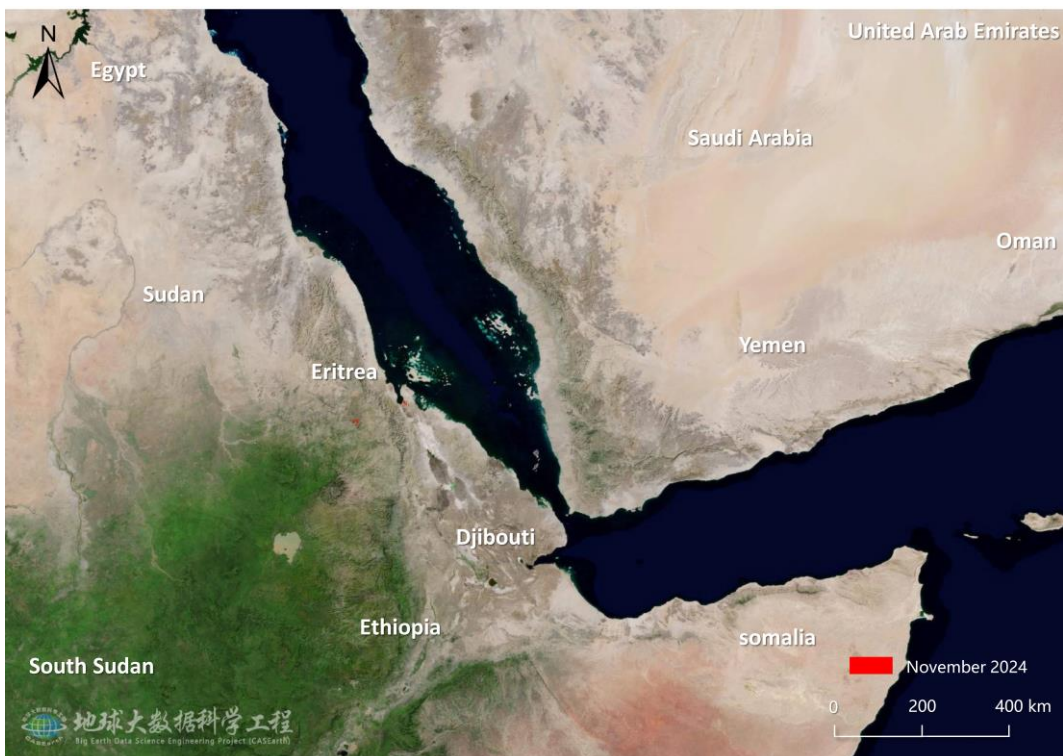
图 1. 厄立特里亚沙漠蝗危害区域遥感监测图（2024 年 11 月）
